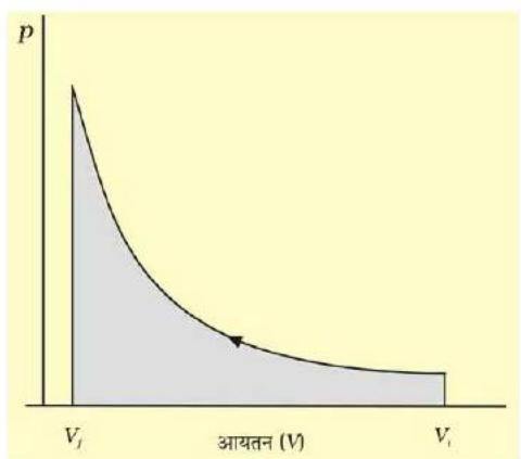
चित्र 6.5 (ग) pV वक्र जब प्रारंभिक आयतन V_i से V_f तक पहुँचने के लिए उत्क्रमणीय परिस्थितियों में लगातार बदलते हुए अस्थिर दाब पर अंततः पदों में किया गया कार्य छायादार क्षेत्र से दर्शाया गया है।
