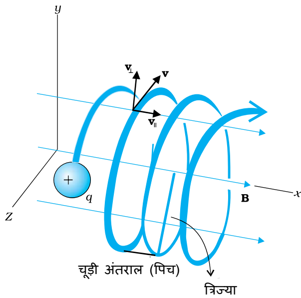
चित्र 4.6 कुंडलिनी गति
