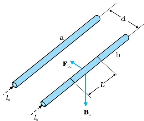
चित्र 4.20 दो लंबे सीधे, समांतर चालक जिनमें अपरिवर्ती धारा i_a एवं i_b प्रवाहित हो रही हैं और जो एक-दूसरे से d दूरी पर रखे हैं। चालक 'a' के कारण चालक 'b' पर उत्पन्न चुंबकीय क्षेत्र B_a है।
