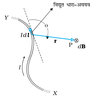
चित्र 4.9 बायो-सावर्ट नियम का निदर्श चित्र। विद्युतधारा-अवयव I dl , r दूरी पर स्थित बिंदु पर क्षेत्र dB उत्पन्न करता है। \otimes चिह्न यह इंगित करता है कि क्षेत्र कागज़ के तल के अभिलंबवत नीचे की ओर प्रभावी है।
