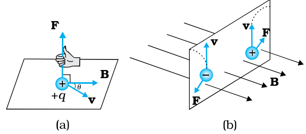
चित्र 4.2 आवेशित कण पर लगे बल की दिशा (a) चुंबकीय क्षेत्र \mathbf{B} से \theta कोण बनाते हुए \mathbf{v} वेग से गतिमान कोई धनावेशित कण बल का अनुभव करता है जिसकी दिशा दक्षिण हस्त नियम द्वारा प्राप्त होती है। (b) चुंबकीय क्षेत्र की उपस्थिति में गतिशील आवेशित कण के विक्षेप q की दिशा -q के विक्षेप की दिशा के विपरीत होती है।
