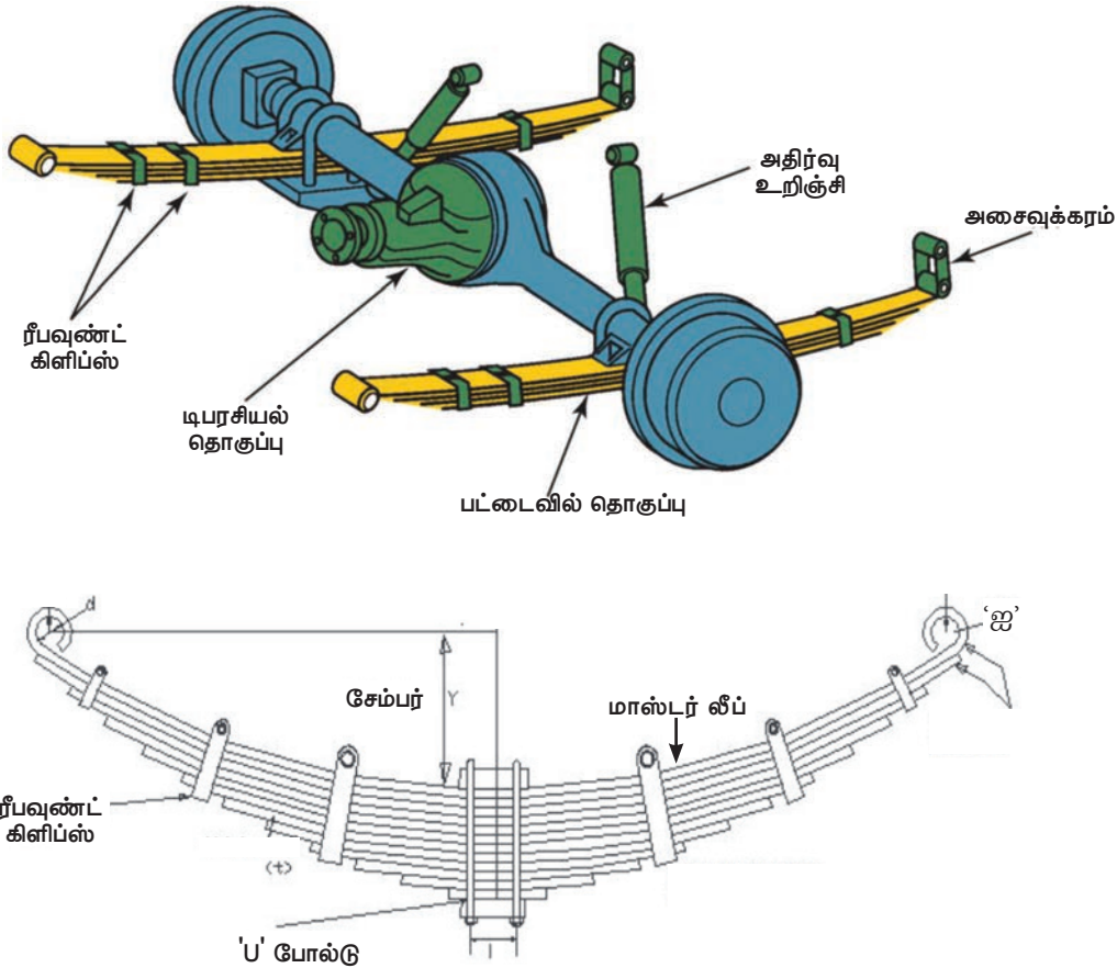
படம் 7.1.1.1 பட்டைவில் தொகுப்பு (Leaf Spring)
