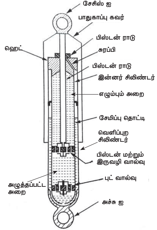
படம் 7.5.2.1 டெலஸ்கோப்பிக் அதிர்வு உறிஞ்சி
