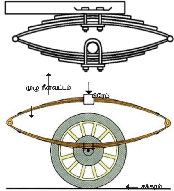
படம் 7.1.1 (ஈ) முழுநீள்வட்ட பட்டைவில்
