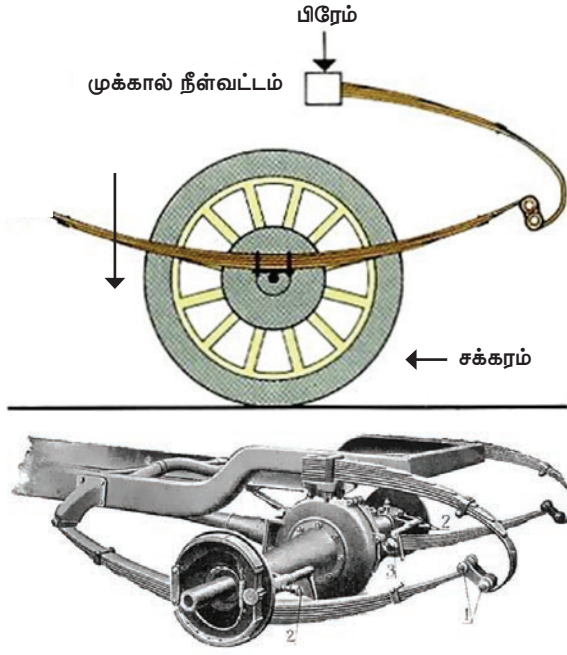
படம் 7.1.1 (இ) முக்கால் நீள்வட்ட பட்டைவில்
