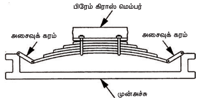
படம் 7.1.1 (உ) குறுக்குவெட்டுபட்டை வில்
