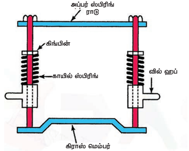
படம் 7.3.2.2 வெர்டிகல் கைடு வகை
