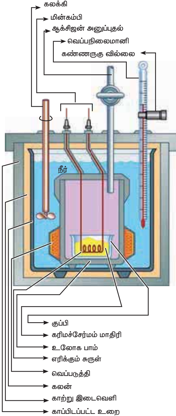
படம் 7.6 பாம் கலோரிமீட்டர்
