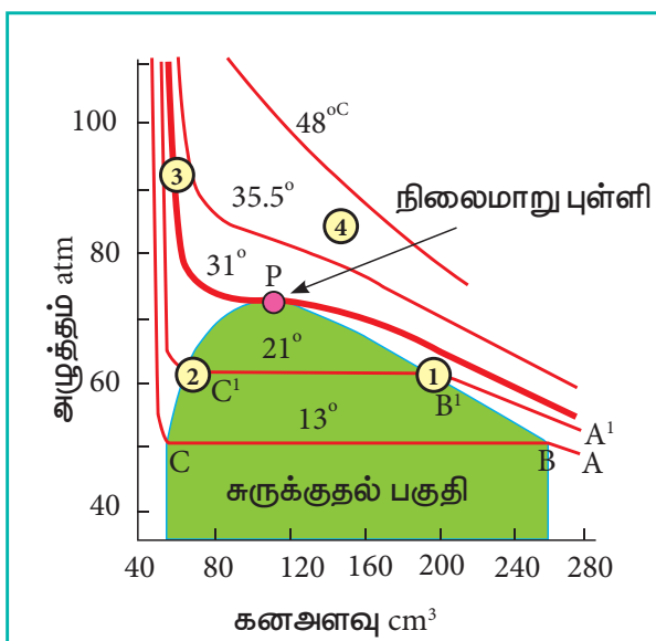
படம் 6.12 வெவ்வேறுவெப்பநிலைகளில் \text{CO}_2 ன் சமவெப்பநிலைக்கோடுகள்
