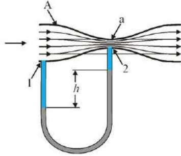
चित्र 10.11 वेंदुरीमापी का व्यवस्था आरेख।
