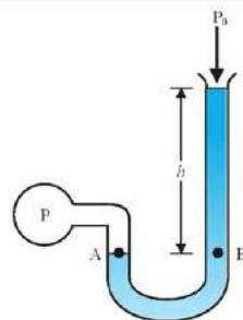
(b) खुली-नली मैनोमीटर (दाबांतर मापी)
