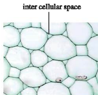
Parenchyma
