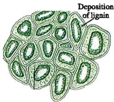
Sclerenchyma
