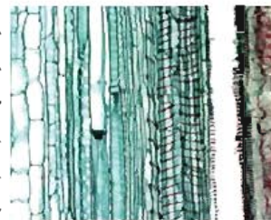
Xylem
