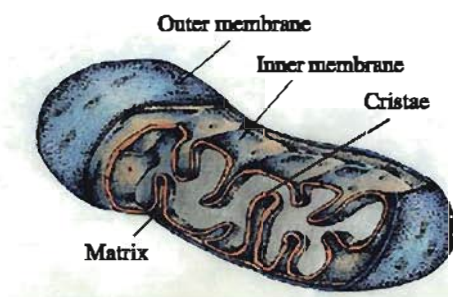
Mitochondria
