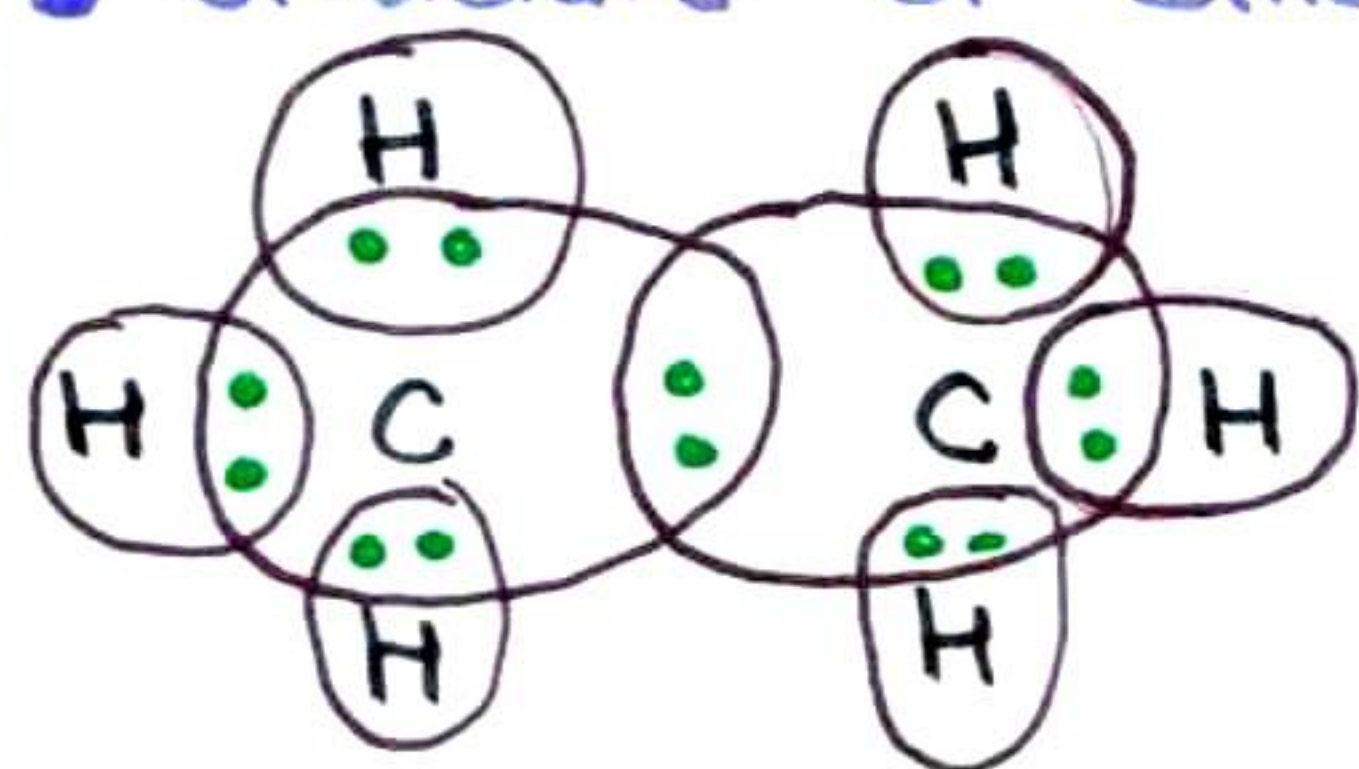
C_2H_6
