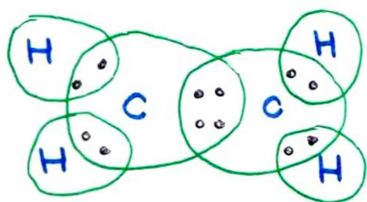
C_2H_4
