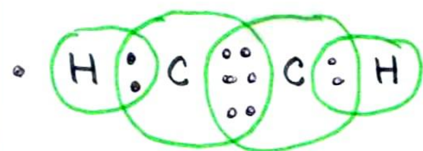
C_2H_2
