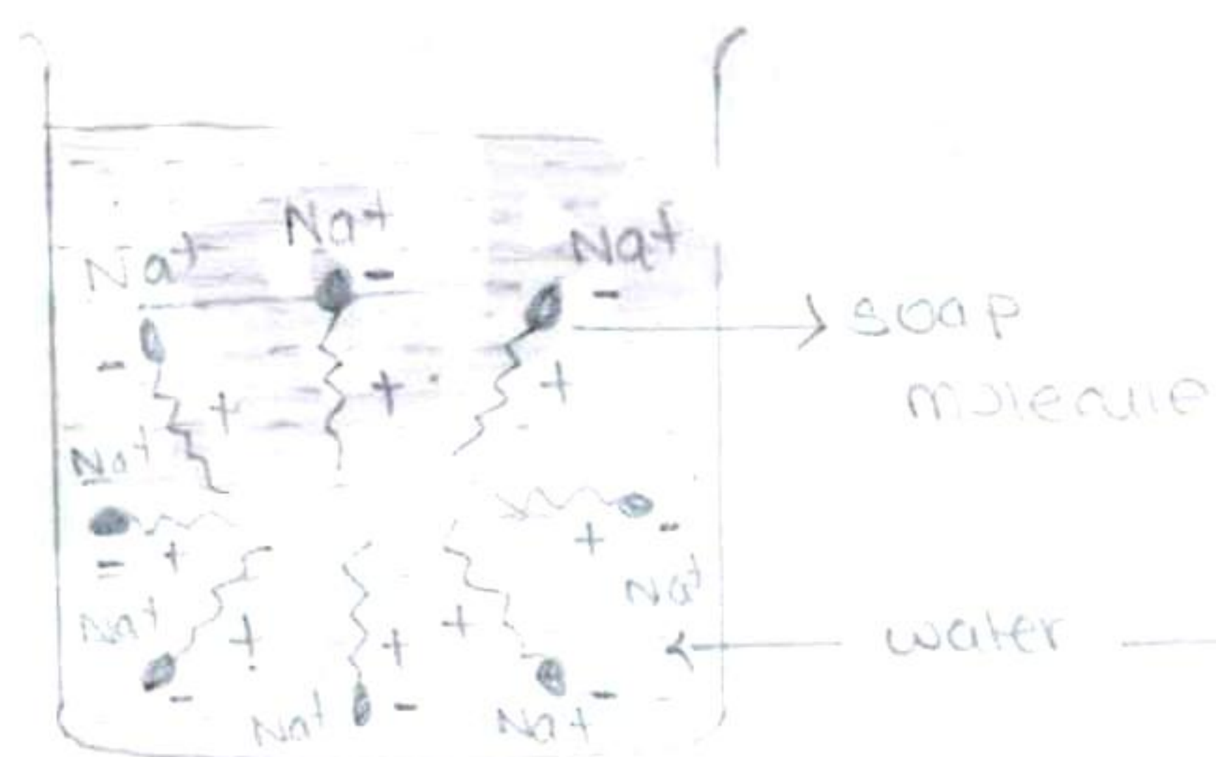
a. Soap micelle
