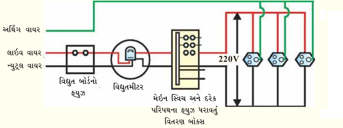
આકૃતિ 13.20 એક સામાન્ય ઘરેલું પરિપથનું રેખાચિત્ર
