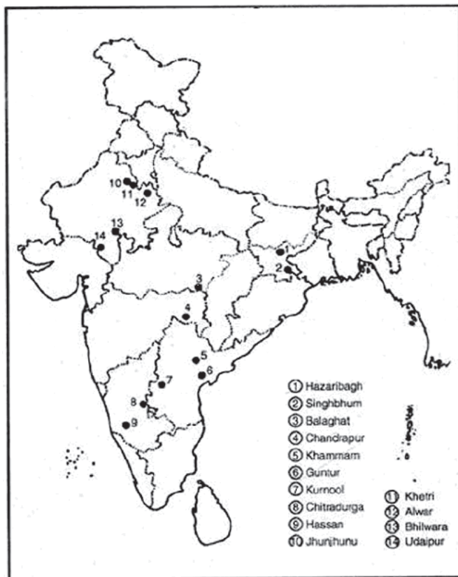
ताम्र निक्षेप
