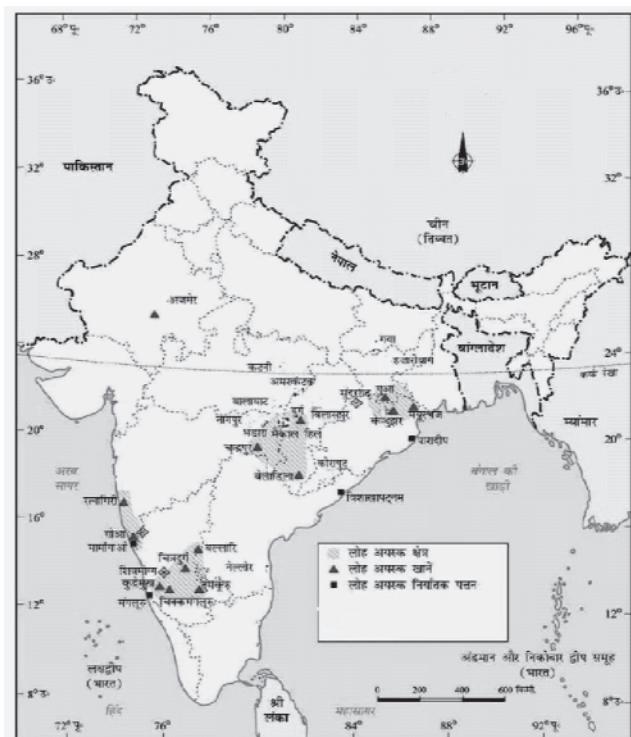
लोहा निक्षेप
