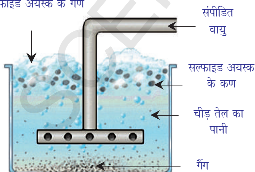
चित्र-1: सल्फाइड अयस्क के लिये झाग-फ्लवन
