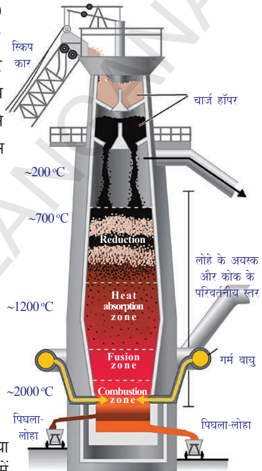
चित्र-6: ब्लास्ट फरनेस
