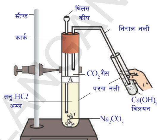
चित्र-2: \text{Ca(OH)}_2 विलयन में \text{CO}_2 गैस को प्रवाहित करना
