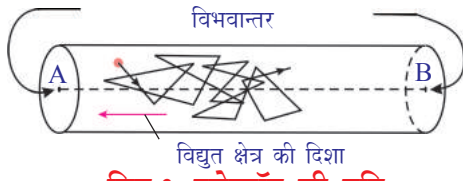
चित्र-3: इलेक्ट्रॉन की गति
