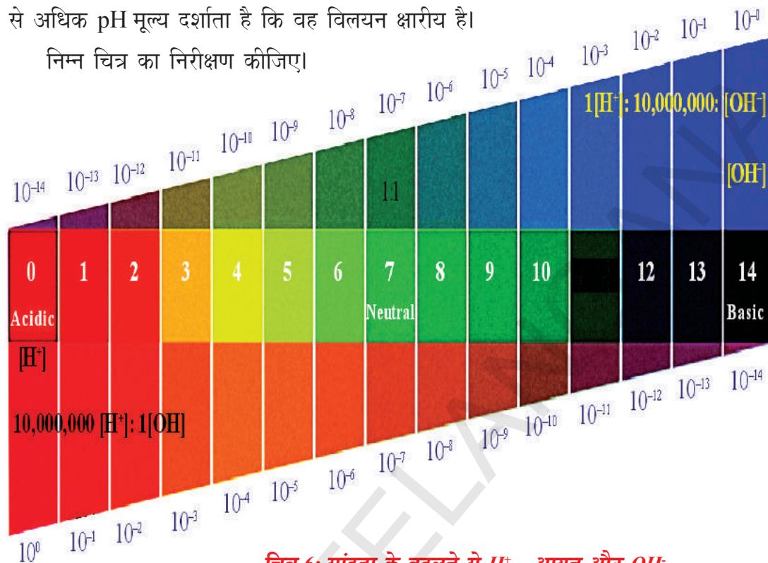
चित्र-6: सांद्रता के बदलने से \text{H}^+_{(aq)} आयन और \text{OH}^-
