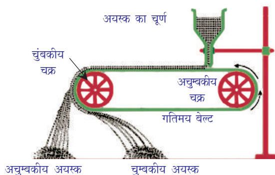
चित्र-2: चुम्बकीय पृथकीकरण
