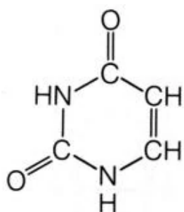
Uracil
