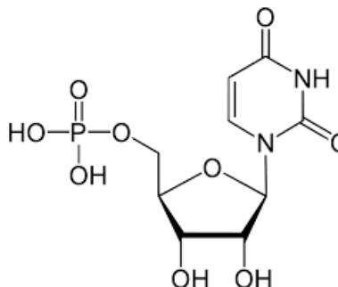
Uridine
