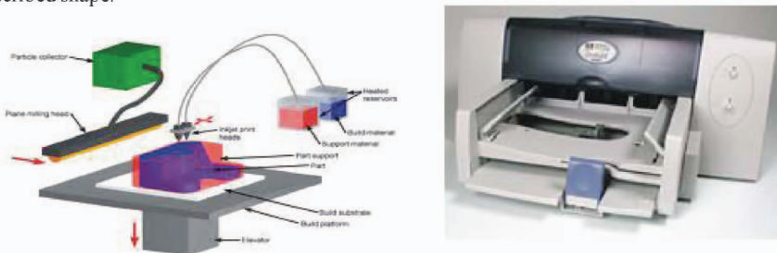
Figure2.15 Inkjet Printer
