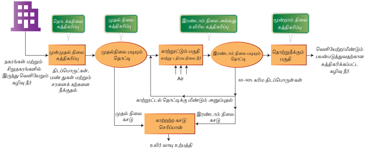
படம் 9.2 கழிவுநீர் சுத்திகரிப்பு முறை
