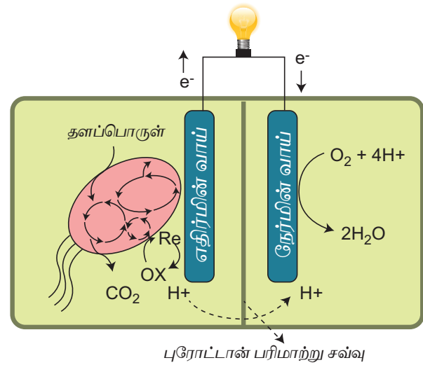
படம் 9.3 நுண்ணுயிரிய எரிபொருள் கலன்
