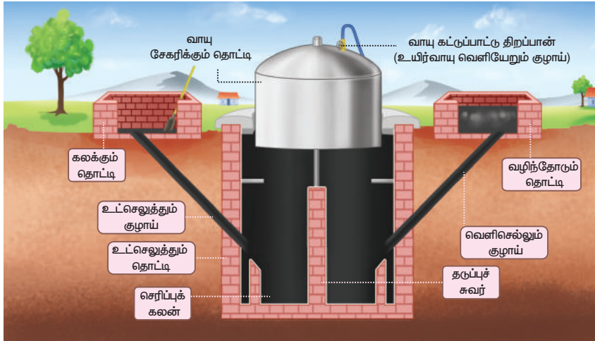
படம் 9.4 உயிர் வாயு அலகு
