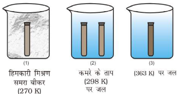
चित्र 7.9 : अभिक्रिया 2\text{NO}_2(g) \rightleftharpoons \text{N}_2\text{O}_4(g) की साम्यावस्था पर ताप का प्रभाव
