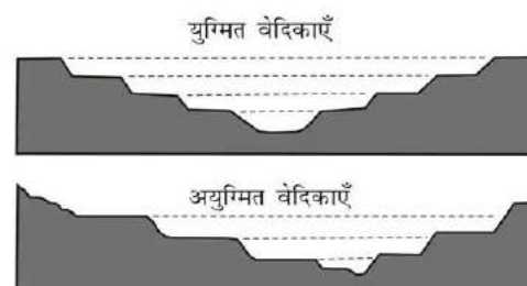
चित्र 7.3 : युग्मित एवं अयुग्मित वेदिकाएँ
