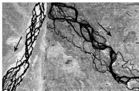
चित्र 7.9 : (बाँयी ओर) गंडक नदी तथा (दाँयी ओर) सोन नदी के गुम्फित प्रणाली खंड दर्शाने वाला उपग्रही चित्र। तीर के चिह्न नदी प्रवाह की दिशा प्रकट करते हैं
