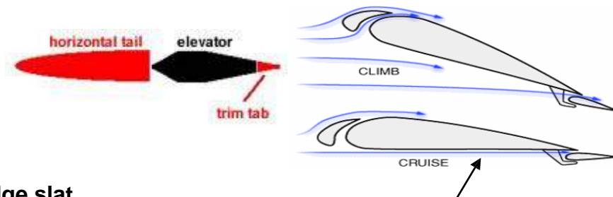
Leading edge slat
