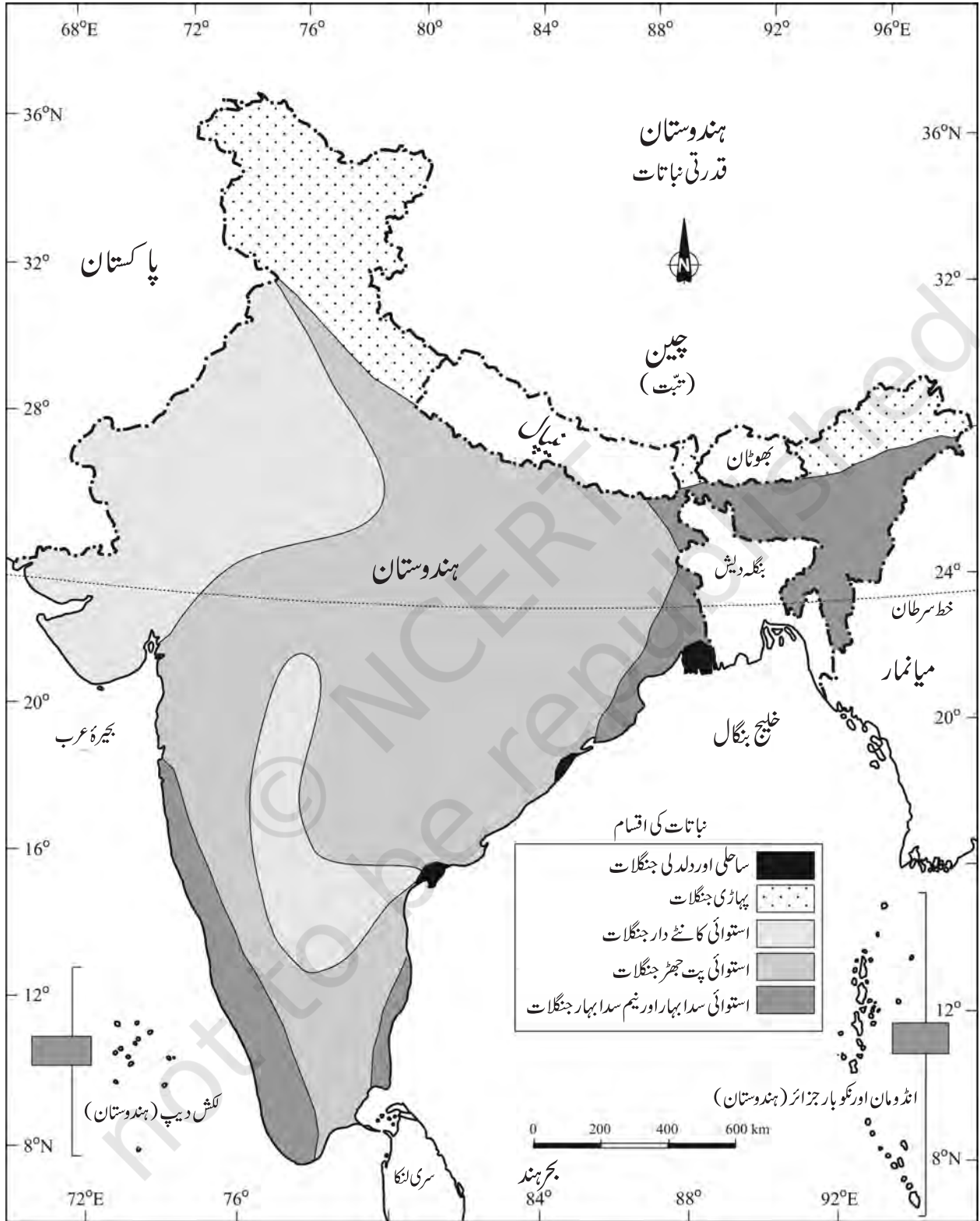
شکل 5.2 : قدرتی نباتات
