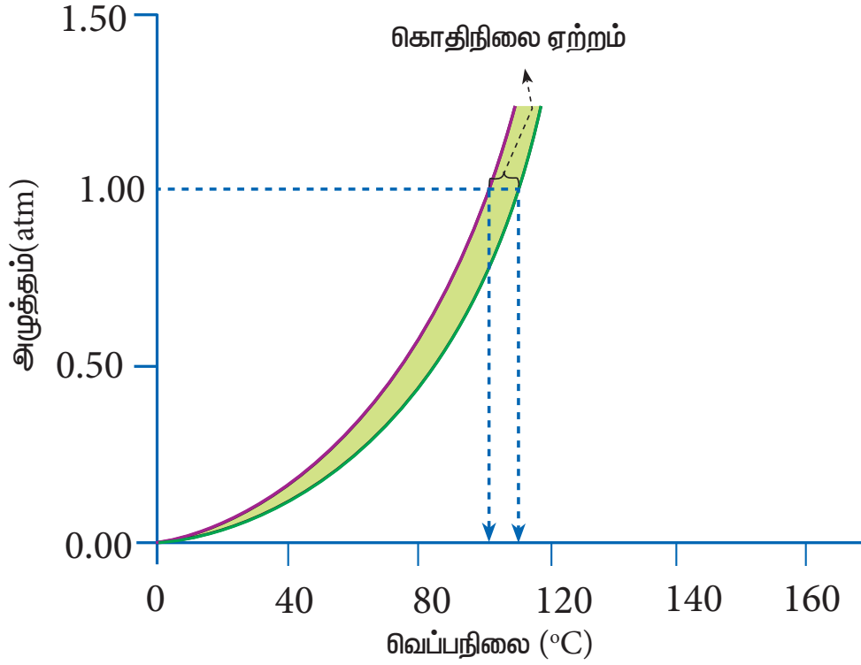
படம் 9.11 கொதிநிலை ஏற்றம்
