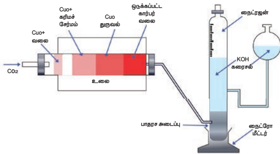
படம் 11.5 டுமாஸ் முறை
