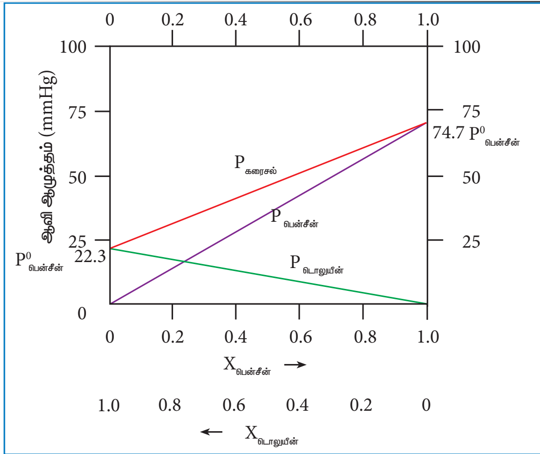
படம் 9.5 டொலுயீனில் கரைந்த பென்சீன் கரைசல் ரௌல்ட் விதிக்கு உட்படுகிறது
