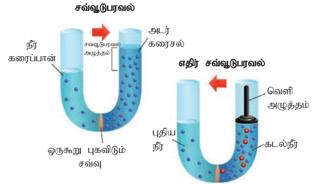
படம் 9.15 சவ்வுப் பரவல் & எதிர்சவ்வுப் பரவல்
