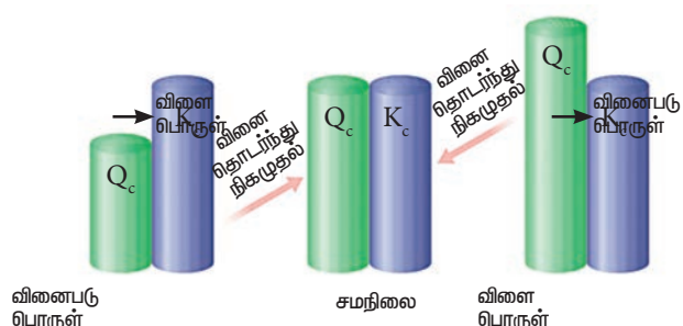
படம் 8.4 வினை நிகழும் திசையினை தீர்மானித்தல்
