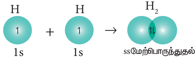
படம் 10.18 ஹைட்ரஜன் மூலக்கூறு உருவாதல்
