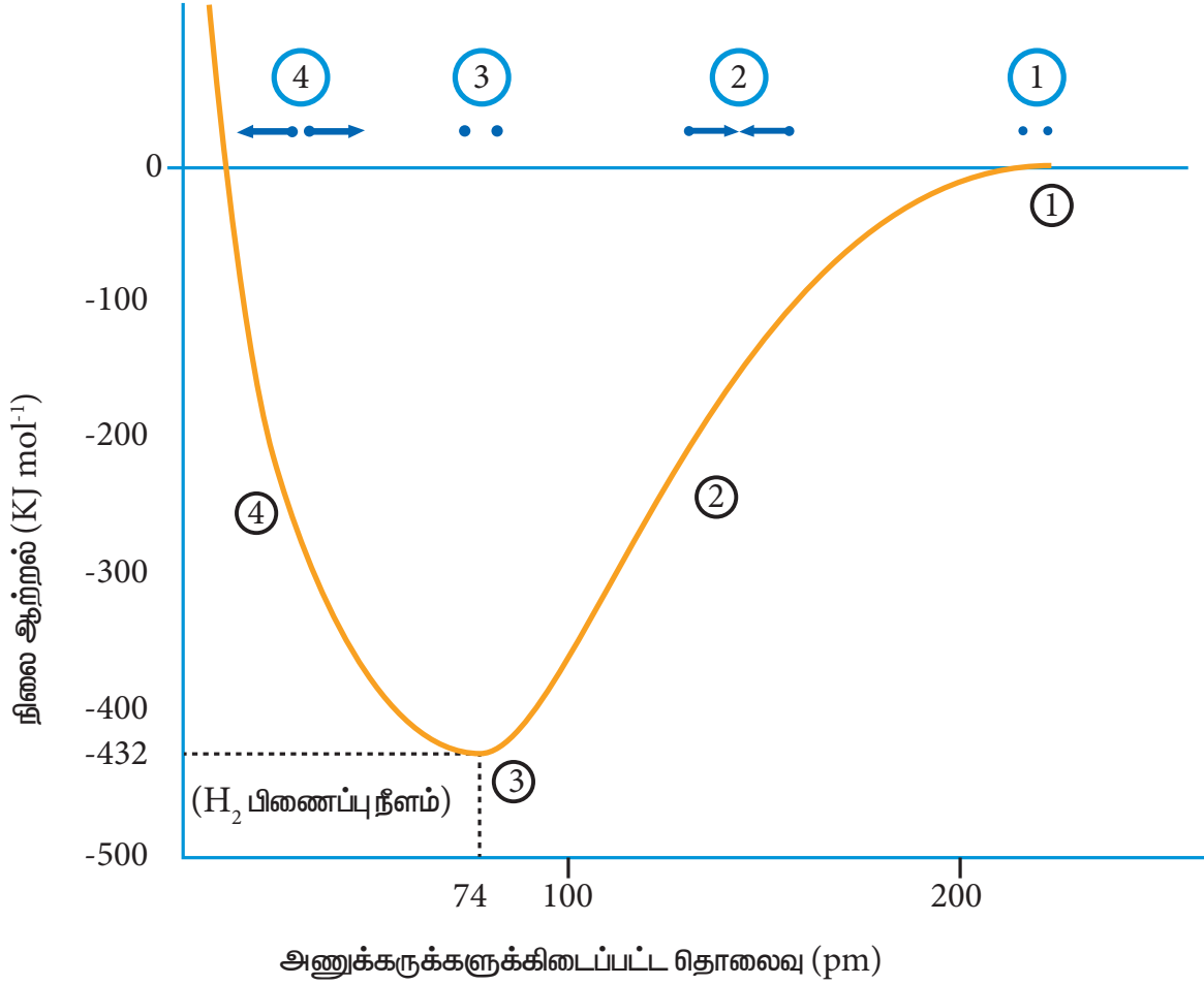
படம் 10.17 (ஆ) H_2 மூலக்கூறு உருவாதல்- VB கொள்கை
