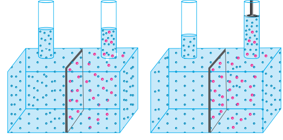
படம் 9.13 சவ்வுடு பரவல் மற்றும் சவ்வுடுபரவல் அழுத்தம்
