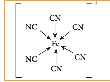
படம் 10.11 பெர்ரோ சயனைடு அயனியின் அமைப்பு
