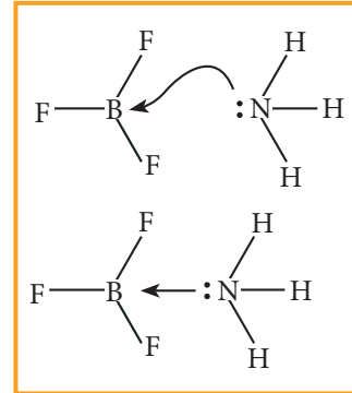
படம் 10.12 BF_3 \rightarrow NH_3 வடிவமைப்பு
