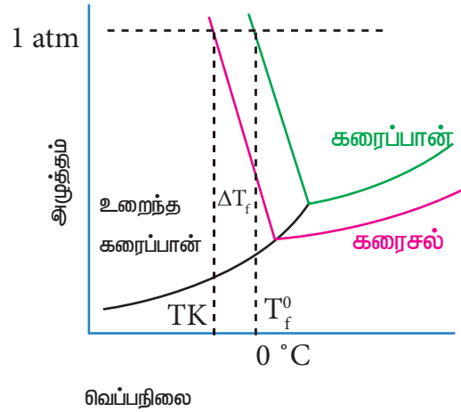
படம் 9.12 உறைநிலைத் தாழ்வு
