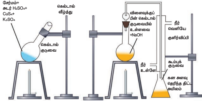
படம் 11.4 கெல்டால் முறை
