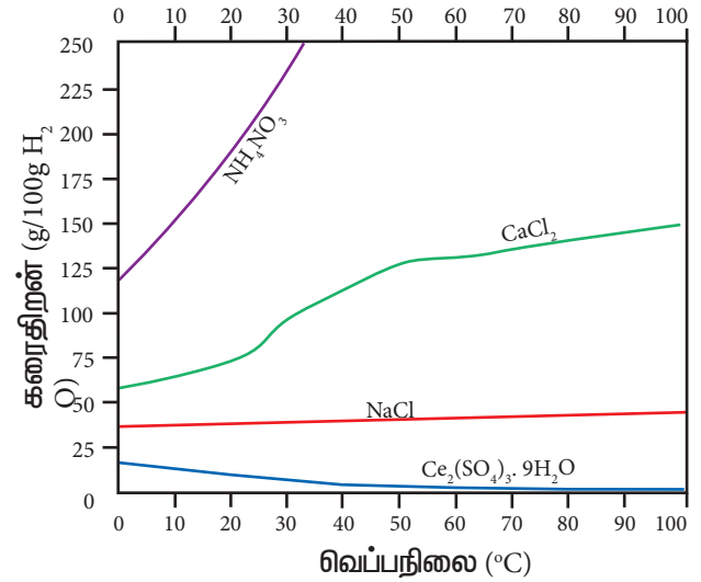
படம் 9. 1 தேர்ந்தெடுக்கப்பட்ட சேர்மங்களின், வெப்பநிலைக்கு எதிரான கரைதிறன் வரைபடம்
