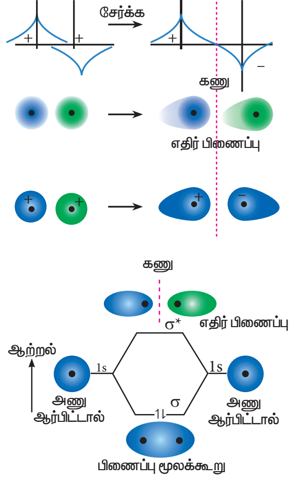
படம் 10.29 அணு ஆர்பிட்டால்களின் நேர்கோட்டு இணைவு
