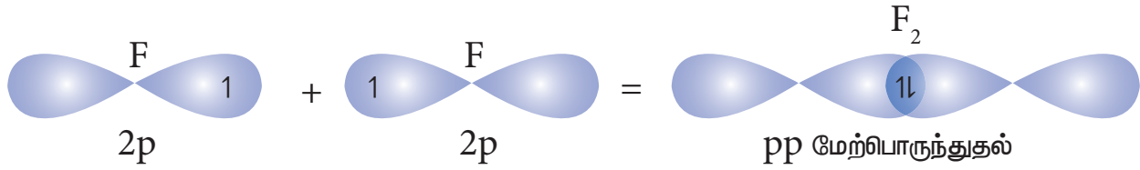
படம் 10.19 F_2 மூலக்கூறு உருவாதல்
