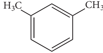
m-சைலீன் 1,3- டைமெத்தில் பென்சீன்
