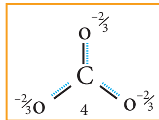
படம் 10. 14 (இ) \text{CO}_3^{2-} அயனியின் உடனிசைவு இனக்கலப்பு அமைப்பு
