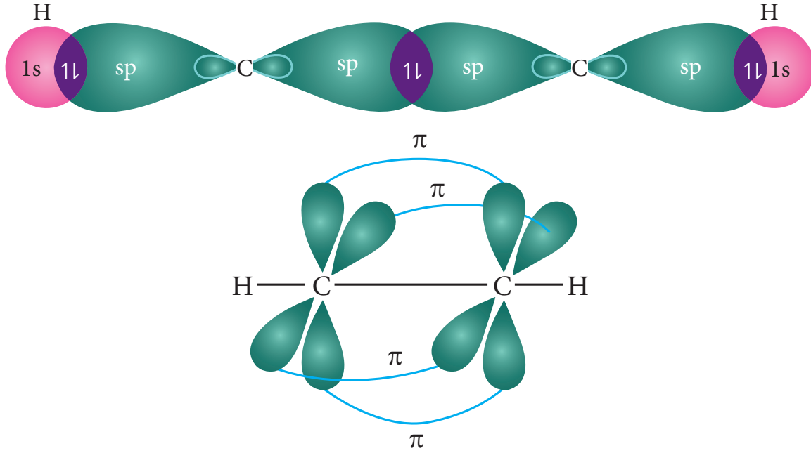
படம் 10.28 அசிட்டிலீனில் sp இனக்கலப்பு
