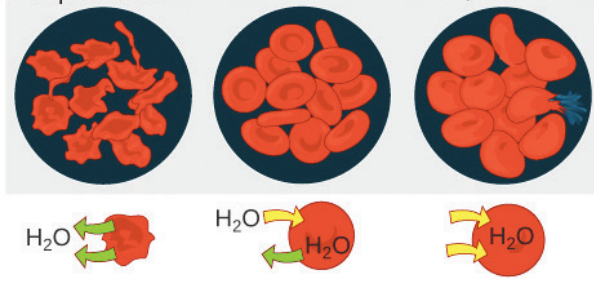
படம் 9. 14 ஐசோடானிக் கரைசல்கள்
