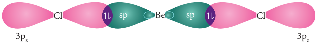
படம் 10.22 sp இனக்கலப்பாதல் : BeCl 2
