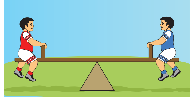
படம் 8.1 சமநிலைக்கான விளக்கப்படம்
