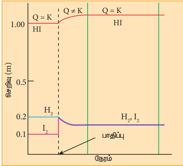
படம் 8.5 அயோடினின் சேர்க்கப்படுவதால் HI உருவாதலில் ஏற்படும் விளைவு.
