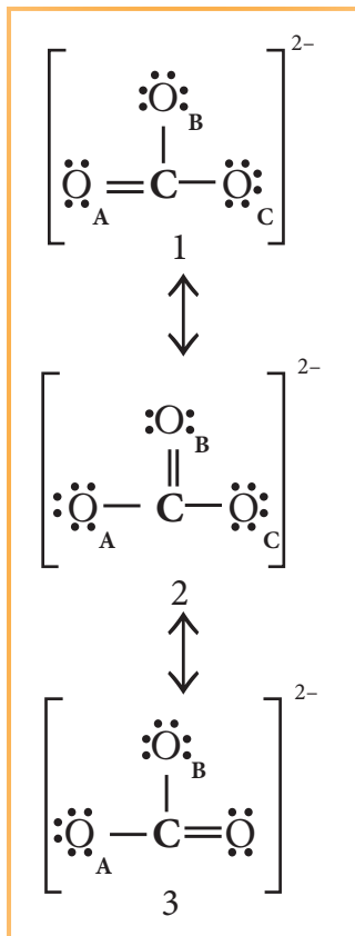
படம் 10. 14 (b) \text{CO}_3^{2-} அயனியின் உடனிசைவு அமைப்புகள்
