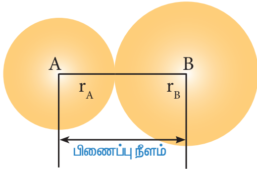
படம் 10.13 A – B சகப்பிணைப்பு மூலக்கூறின் பிணைப்பு நீளம்
