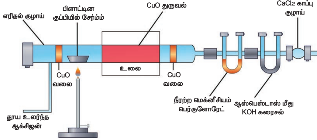
படம் 11.3 கார்பன் மற்றும் ஹைட்ரஜனை எடையறிதல்
