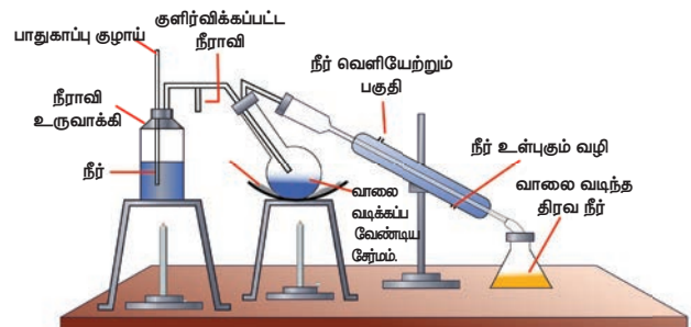
படம் 11.2 நீராவி வாலை வடித்தல்
