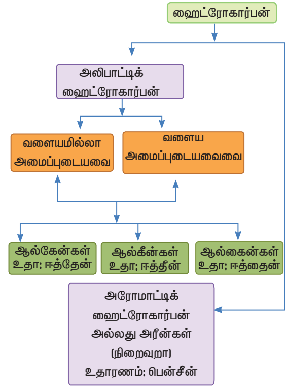
படம் 13.1. ஹைட்ரோகார்பன்களின் வகைகள்
