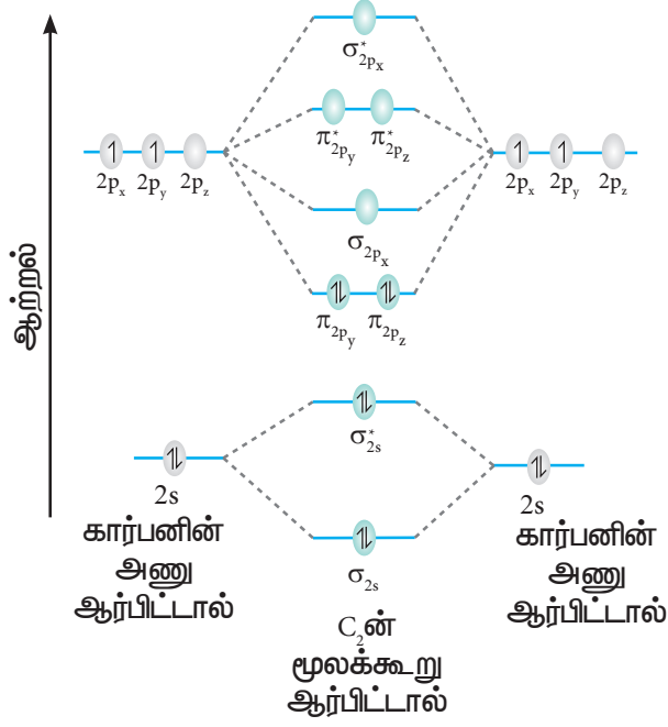
படம் 10.33. கார்பன் ( C_2 ) மூலக்கூறு ஆர்பிட்டால் வரைபடம்
