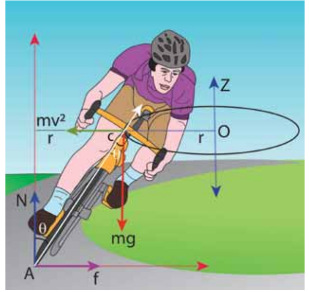
படம் 5.19 வட்டப்பாதையில் சைக்கிள் ஒட்டுபவரின் இயக்கம்
