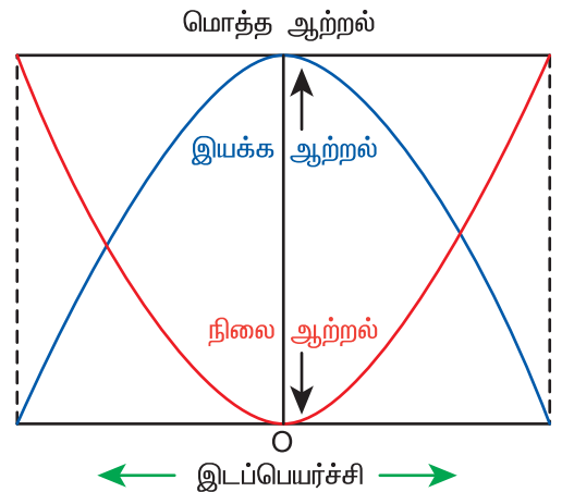
படம் 4.11 சுருள்வில் – நிறை அமைப்பின் நிலை ஆற்றல் – இடப்பெயர்ச்சி வரைபடம்.
