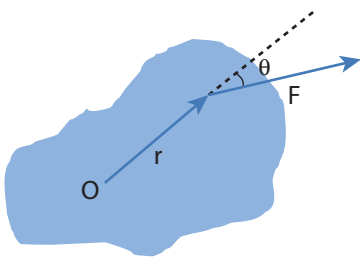
படம் 5.4 ஒரு திண்மப்பொருளின் மீதான திருப்புவிசை
