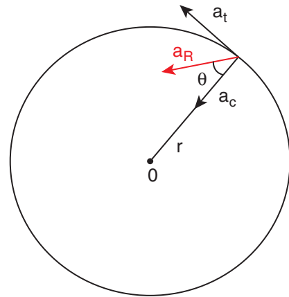
படம் 2.53 சீரற்ற வட்ட இயக்கத்தில் தொகுபயன் முருக்கம் a_R
