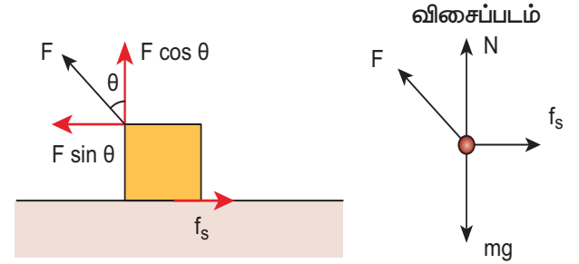
படம் 3.27 பொருளொன்றை \theta கோணத்தில் இழுத்தல்
