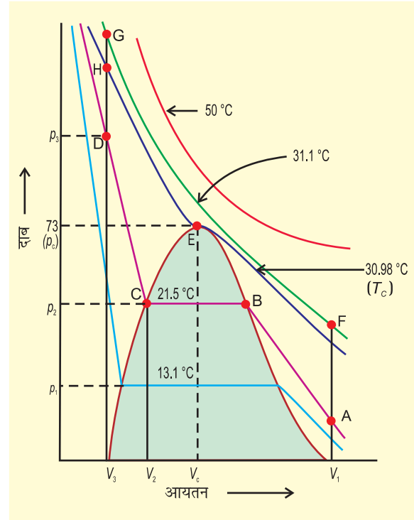
चित्र 5.13: विभिन्न तापों पर कार्बन डाइऑक्साइड के समतापी आरेख
