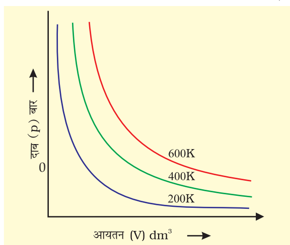
चित्र 5.5 (अ) विभिन्न तापों पर एक गैस के आयतन V के p मध्य वक्र
