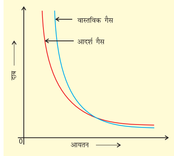
चित्र 5.11 आदर्श गैस तथा वास्तविक गैस के लिए दाब-
