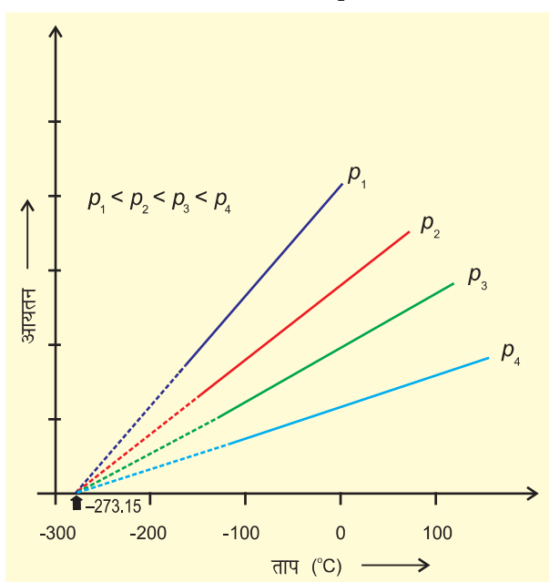
चित्र 5.6 आयतन एवं ताप (°C) के मध्य आरेख
