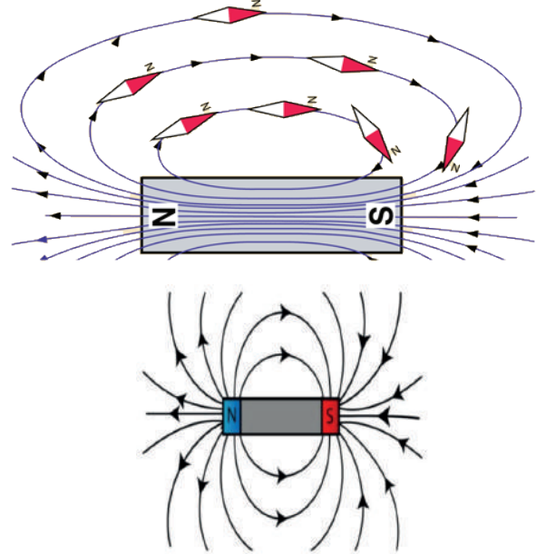
படம் 7.4 காந்தப்புலம்
