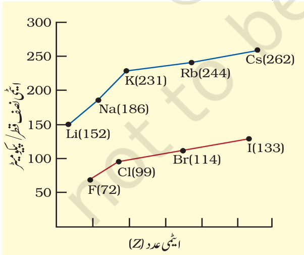
شکل 3.4(b) قلوبی دھاتوں اور ہیلوجنوں کے لیے ایٹمی عدد کے ساتھ ایٹمی نصف قطر میں تغیر۔
