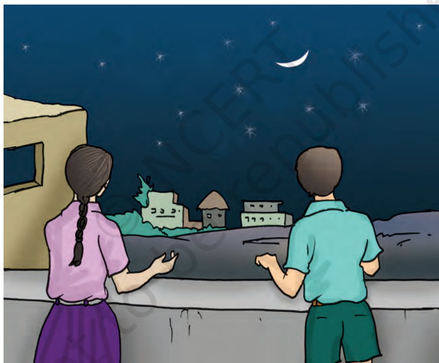
Fig. 17.1: Night sky
