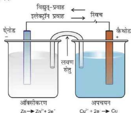
चित्र 8.3 डैनिश सेल की आयोजना। ऍनोड पर Zn के ऑक्सीकरण द्वारा उत्पन्न इलेक्ट्रॉन बाहरी परिपथ से कैथोड तक पहुँचते हैं। सेल के अंदर का परिपथ लवण-सेतु के माध्यम से आयनों के विस्थापन द्वारा पूरा होता है। ध्यान दीजिए कि विद्युत्-प्रवाह की दिशा इलेक्ट्रॉनों के प्रवाह की दिशा के विपरीत है।
