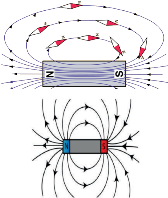
படம் 2.4 காந்தப்புலம்
