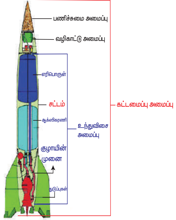
படம் 3.1 ராக்கெட்டின் பகுதிகள்
