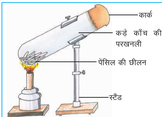
चित्र 6.2 लकड़ी का चारकोल बनाना
