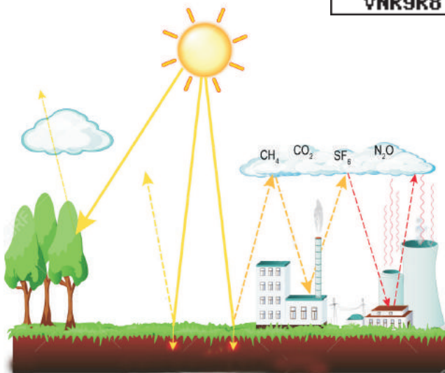
चित्र 3.4 पौधाघर प्रभाव
