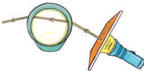
चित्र 9.1 माध्यम परिवर्तन के कारण प्रकाश का मुड़ना
