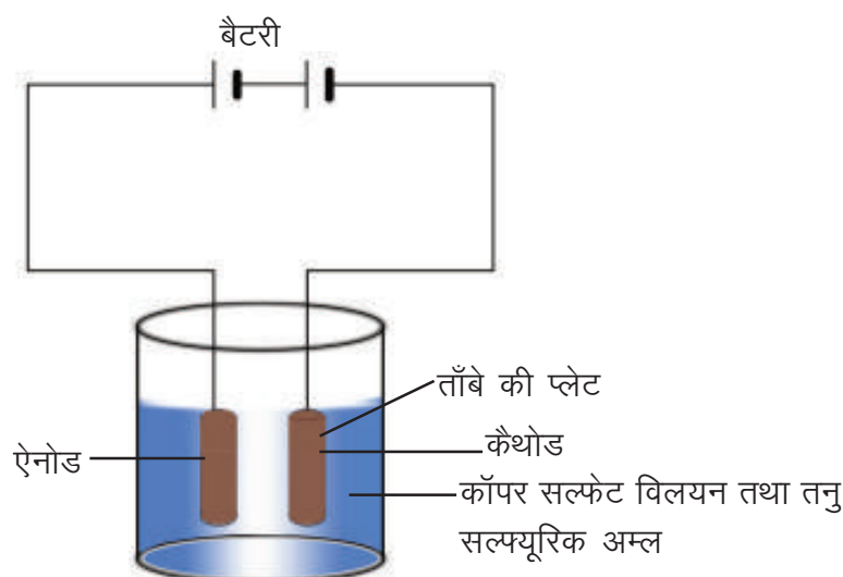
चित्र-11.5 विद्युत लेपन
