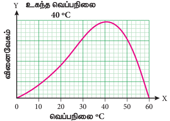
படம் 10.6 வினைவேகம் Vs வெப்பநிலை
