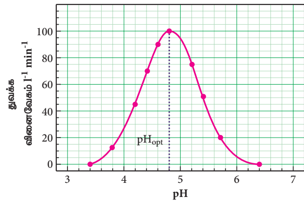
படம் 10.7 வினைவேகம் vs pH
