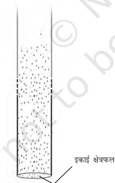
चित्र 11.17 : इकाई क्षेत्रफल के वायुस्तम्भ पर लगने वाला गुरुत्व बल वायुमंडलीय दाब के बराबर है।
