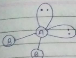
Bent
