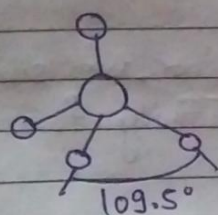
CH 4
