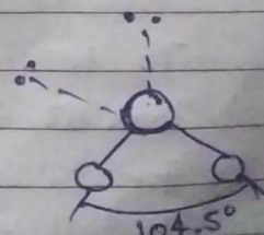
H 2 O
