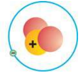
ట్రీటియం {}_1\text{H}^3
