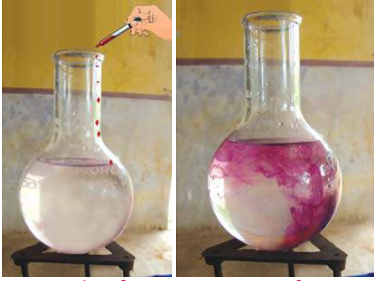
పటం-6 : నీటిలో పోటాషియం పర్మాంగనేట్ వ్యాపనం
