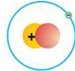
డ్యూటీరియం {}_1\text{H}^2
