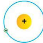
హైడ్రోజన్
