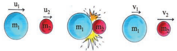
పటం-20 : ద్రవ్యవేగ నిత్యత్వం
