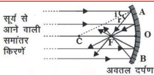
चित्र 14.11 अवतल दर्पण की अभिसारी प्रकृति
