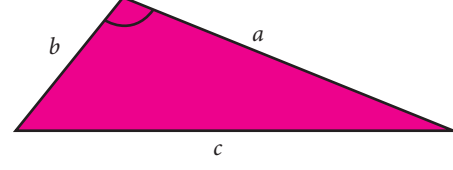
விரிகோண முக்கோணம்
