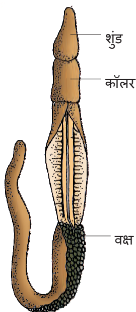
चित्र 4.15 बैलैनोग्लोसस
