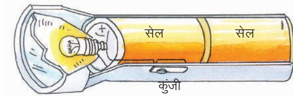
चित्र 21.2 ग टॉर्च का विद्युत परिपथ
