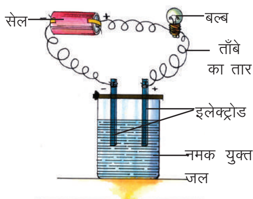
चित्र-2.3 विद्युत चालकता
