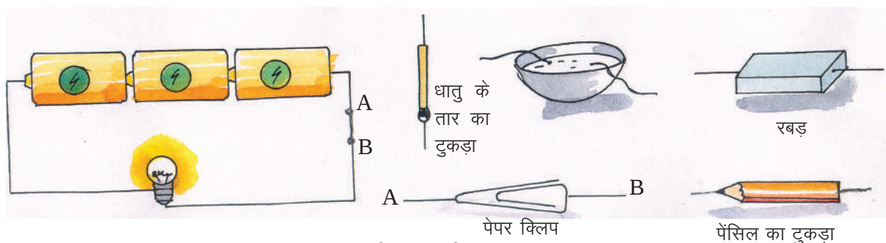
चित्र 21.3 विद्युत सुचालक या हीन चालक पदार्थ
