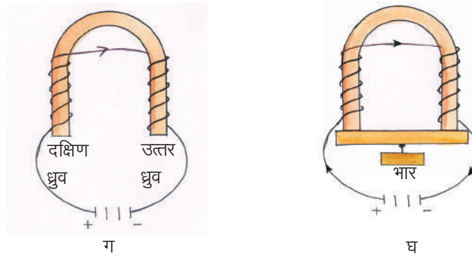
21.8 ग,घ U आकार के लोहे से विद्युत चुंबक बनाना
