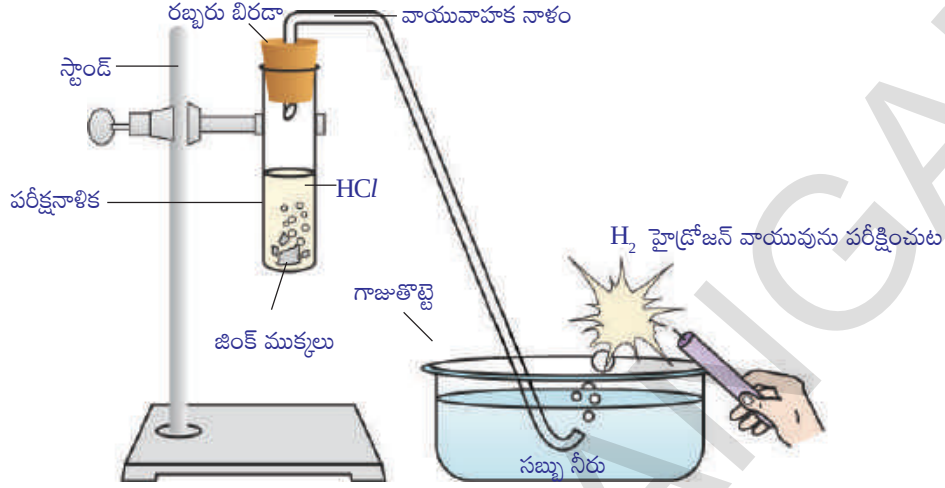
పటం-1 విలీన HCl తో జింక్ ముక్కల చర్య మరియు మండుతున్న కొవ్వొత్తితో హైడ్రోజన్ వాయువును పరీక్షించుట
