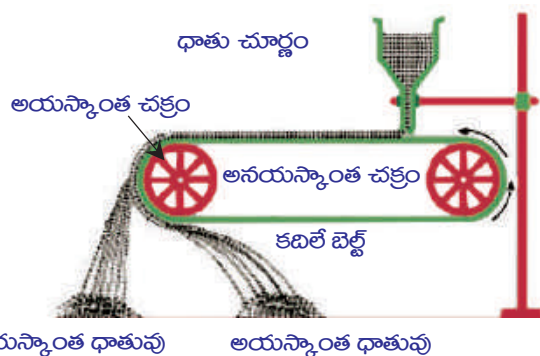
పటం-2 : అయస్కాంత వేర్పాటు పద్ధతి
