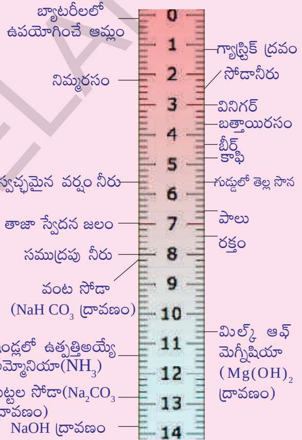
పటం-8 : pH స్కేల్పై ద్రావణాల స్థానం
