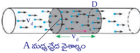
పటం-4: ధనావేశాల డ్రీఫ్ట్
