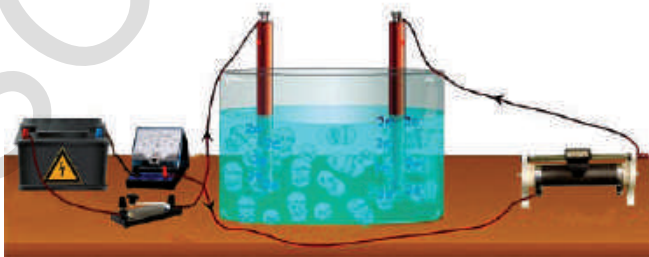
పటం 4 : కాపర్ యొక్క విద్యుత్ శోధన కొరకు పరికరాల అమరిక
