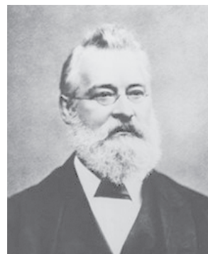
న్యూలాండ్స్
