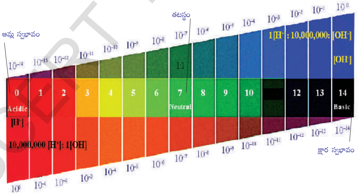
పటం- 6: \text{H}^+ , \text{OH}^- అయాన్ల గాఢతలోని మార్పుతో మారే pH విలువలు
