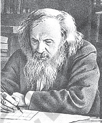
మెండలీఫ్
