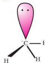
चित्र 12.3 (ख) मेथिल कार्बऋणायन (carbanion) की आकृति
