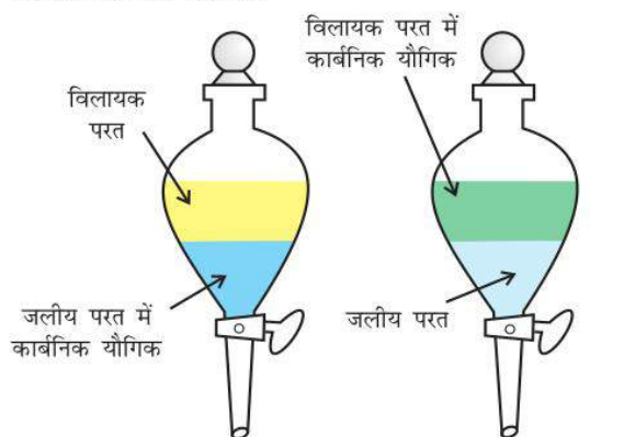
निष्कर्षण से पहले निष्कर्षण के पश्चात् चित्र 12.10 विभेदी निष्कर्षण। अवयवों का पृथक्करण विलेयता में अंतर पर आधारित होता है।
