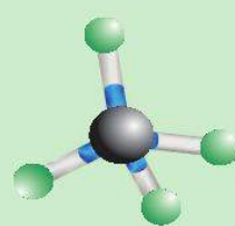
बॉल एवं स्टिक मॉडल
