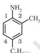
4-एथिल-2-मेथिलएनीलीन
