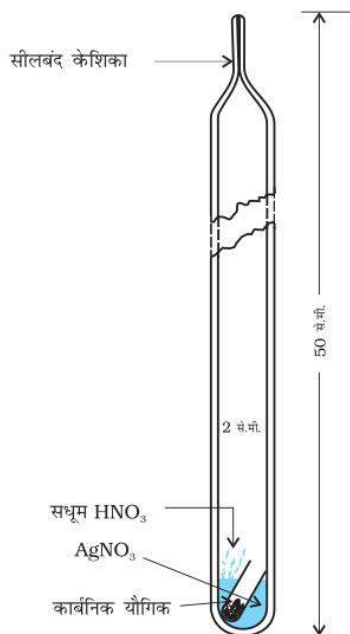
चित्र 12.17 कैरीयस विधि-हैलोजनयुक्त कार्बनिक यौगिक को सिल्वर नाइट्रेट की उपस्थिति में संथूम नाइट्रिक अम्ल के साथ गरम किया जाता है।
