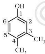
3, 4-डाइमेथिलफीनॉल
