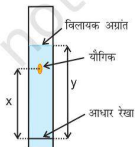
चित्र 12.12 (ख) विकसित क्रोमेटोग्राम
