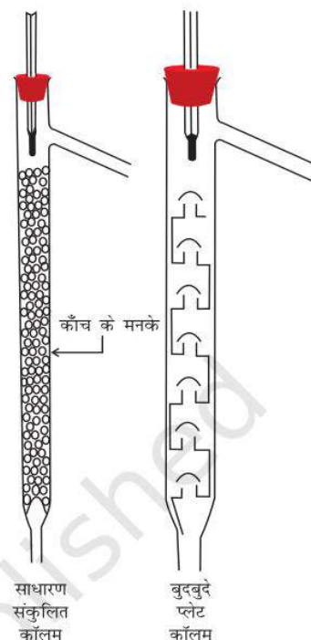
चित्र 12.7 विभिन्न प्रकार के प्रभाजी कॉलम
