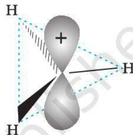
चित्र 12.3 (क) मेथिल कार्बधनायन की आकृति
