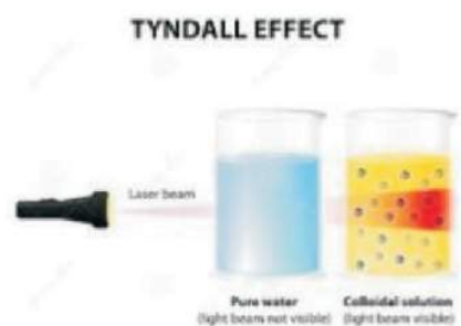
चित्र-3.2 टिण्डल प्रभाव
