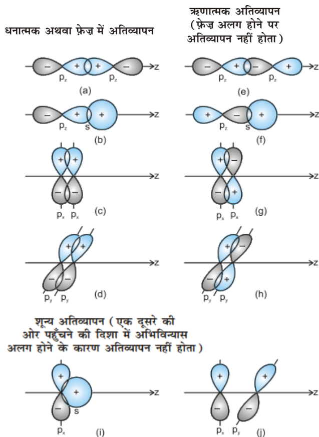
चित्र 4.9 s तथा p परमाणु कक्षकों के धनात्मक, ऋणात्मक तथा शून्य अतिव्यापन
