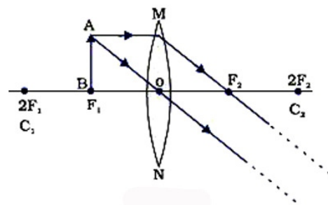
Fig 9.31 (d) Object at F_1
