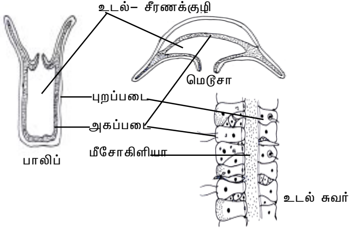
படம் 1.2.4 குழியுடலி - உடல் சுவர்
