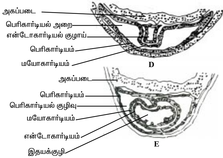
படம்.5.1.14. தவளையின் கருவில் இதயம் தோன்றுதல்
