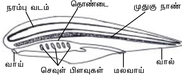
படம். 1.2.17 முதுகு நாணிகள் - ஓர் விளக்கப்படம்
