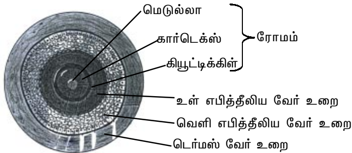
படம்.3.1.3. பாலிக்கின் பகுதியில் ரோமத்தின் கு. வெ. தோற்றம்
