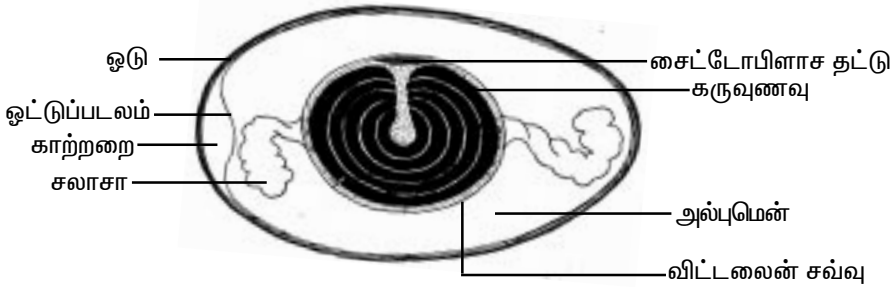
படம்.5.1.2. கோழி முட்டை
