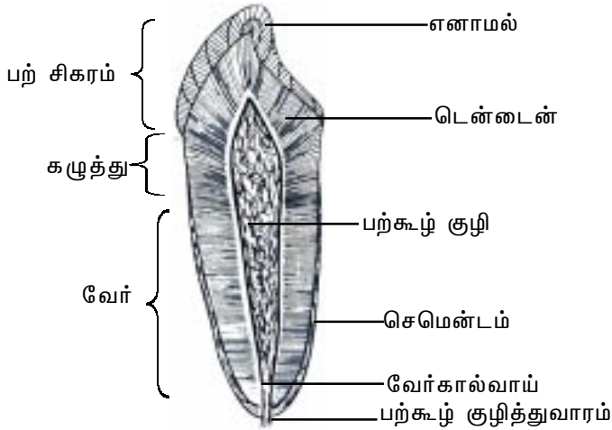
படம்.3.4.3. ஓர் பல்லின் அமைப்பு
