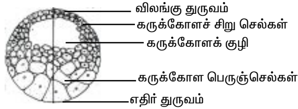
படம்.5.1.7. தவணையின் கருக்கோளம் – வெட்டுத் தோற்றம்
