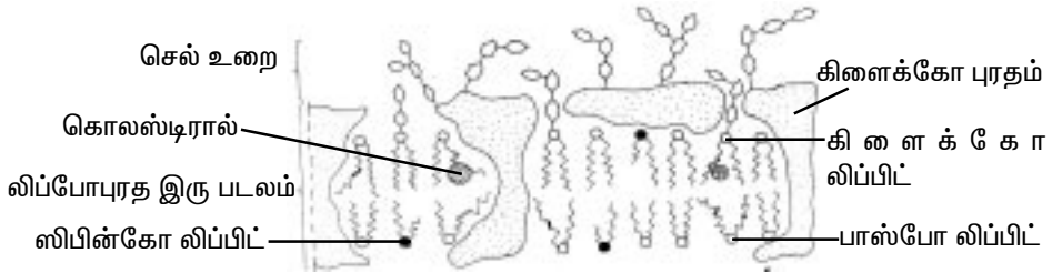
படம்.2.2.2. திரவத்தன்மை கூட்டமைப்பு மாதிரி செல் படலம்
