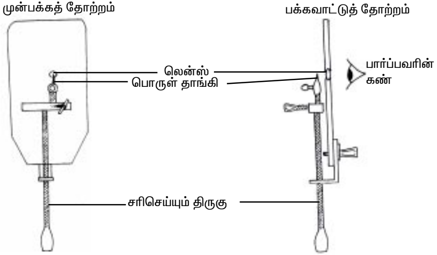
படம்.2.1.1. வான் லீவன் ஹாக்கின் எளிய நுண்ணோக்கி
