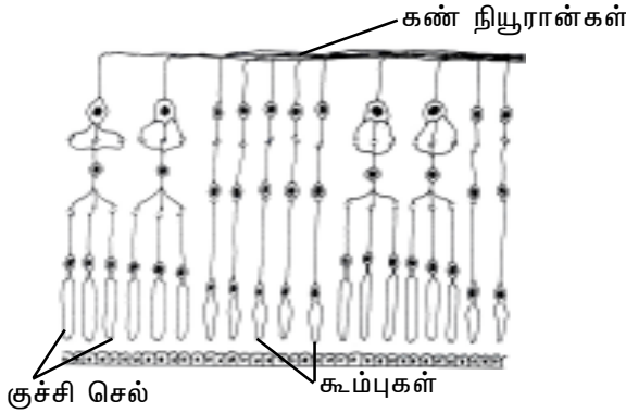
படம். 3.9.3 விழித்திரை - கூம்புகளும் குச்சிகளும்
