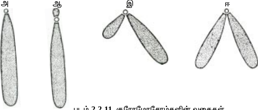
படம்.2.2.11. குரோமோசோம்களின் வகைகள்
