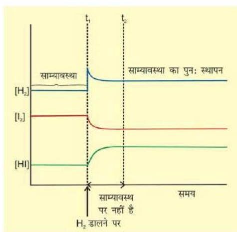
चित्र 7.8 H_2(g) + I_2(g) \rightleftharpoons 2HI(g) अभिक्रिया में साम्यावस्था पर H_2 के डालने पर अधिकारकों एवं उत्पादों के सांद्रण में परिवर्तन
