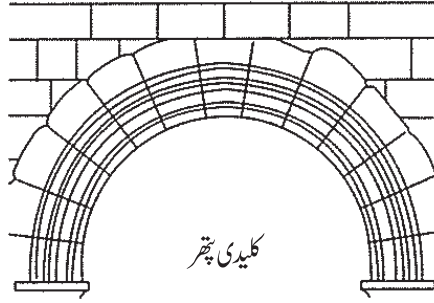
شکل 5a ایک سچی محراب مرکز میں کلیدی پتھر بالائی عمارت کے بوجھ کو محراب کی بنیاد کو منتقل کرتا ہے۔
