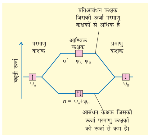
चित्र 4.19 दो परमाणु क्रमशः A तथा B पर केंद्रित परमाणु कक्षकों \psi_A तथा \psi_B के रैखिक संयोग से आबंधन ( \sigma ) तथा प्रतिबंधन ( \sigma^* ) आण्विक कक्षकों का निर्माण।
