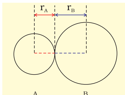
चित्र 4.1: सहसंयोजी अणु AB में आबंध लम्बाई
