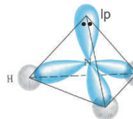
चित्र 4.13 NH_3 अणु का बनना
