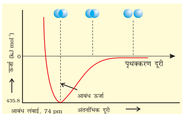
चित्र 4.8: H_2 अणु के विरचन के लिए H परमाणुओं के बीच अंतराणु दूरी की सापेक्ष स्थितिज ऊर्जा का आरेख, आरेख में न्यूनतम ऊर्जा स्थिति H_2 की सर्वाधिक स्थाई अवस्था दर्शाती है।
