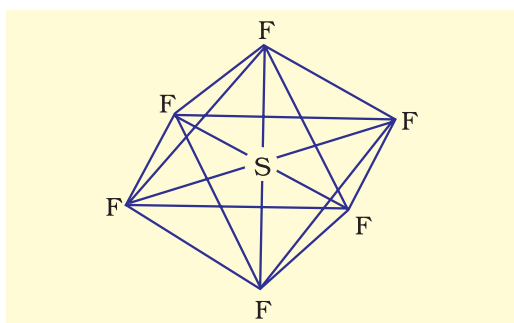
चित्र 4.18 SF_6 अणु की अणु की अष्टफलकीय ज्यामिति
