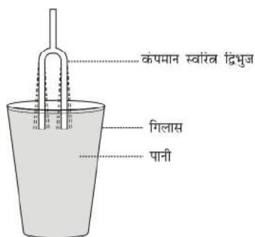
चित्र 12.3: कंपमान स्वरित्र द्विभुज की दोनों भुजाएँ पानी में डूबी हुई
