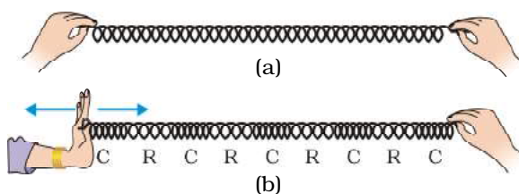
चित्र 12.7: स्प्रिंग में अनुदैर्घ्य तरंग
