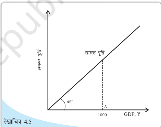
45° लाइन के साथ समस्त पूर्ति वक्र
