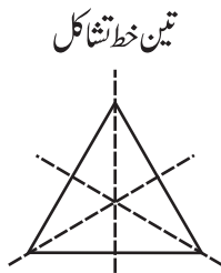
مساوی ضلعی مثلث (i)
