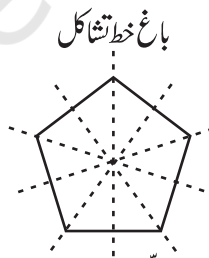
منظم پانچ ضلعی (iii)
