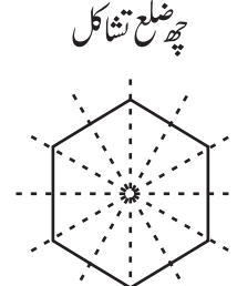
منظم چھ ضلعی (iv)
