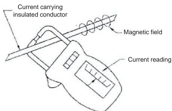
Fig. 6.13 Tong tester
