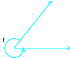
(v) 180^\circ < t < 360^\circ زاویہ معکوس
