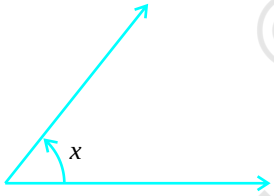
(i) 0^\circ < x < 90^\circ زاویہ حادہ
