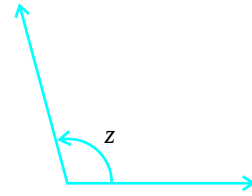
(iii) 90^\circ < z < 180^\circ زاویہ منفرجہ
