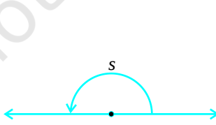
(iv) s = 180^\circ زاویہ مستقیم
