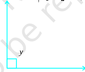
(ii) y = 90^\circ زاویہ قائمہ
