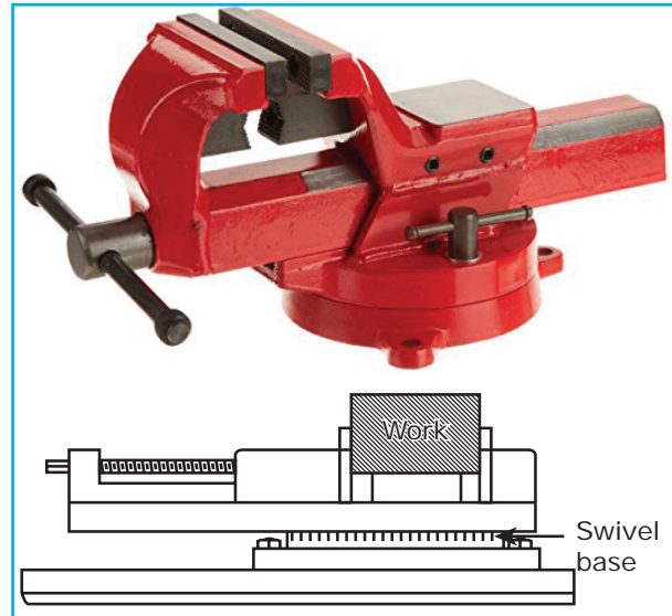
Swivel Vise
