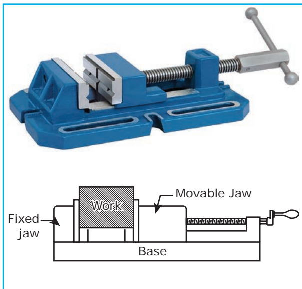
Plain Vise
