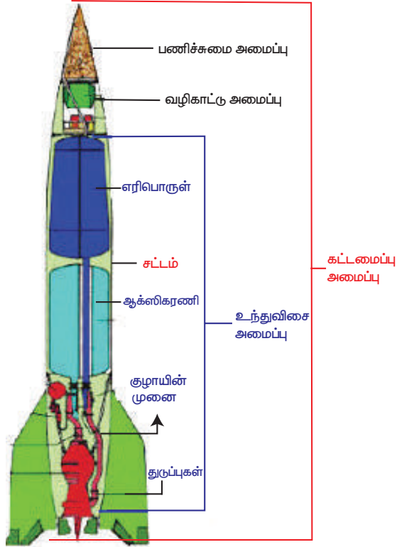
படம் 8.1 ராக்கெட்டின் பகுதிகள்
