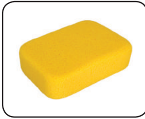
பாலியூரித்தீன்கள்
